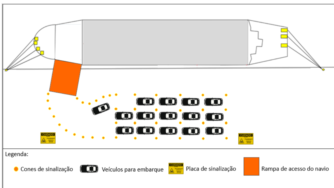
Figura 7 - Esquema ilustrativo de sinalização de segurança e demarcação da área de operação, disposição das filas e rota que os veículos irão percorrer até o navio
