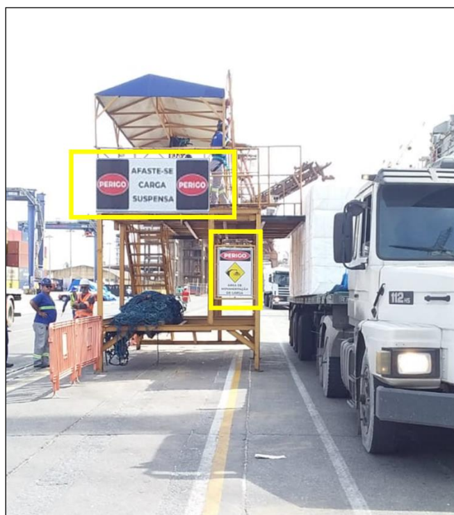
Figura 4 - Ilustração de sinalização de segurança nas plataformas de trabalho em altura, com os dizeres: PERIGO, AFASTE-SE CARGA SUSPensa e AFASTE-SE MOVIMENTAÇÃO DE CARGA.
