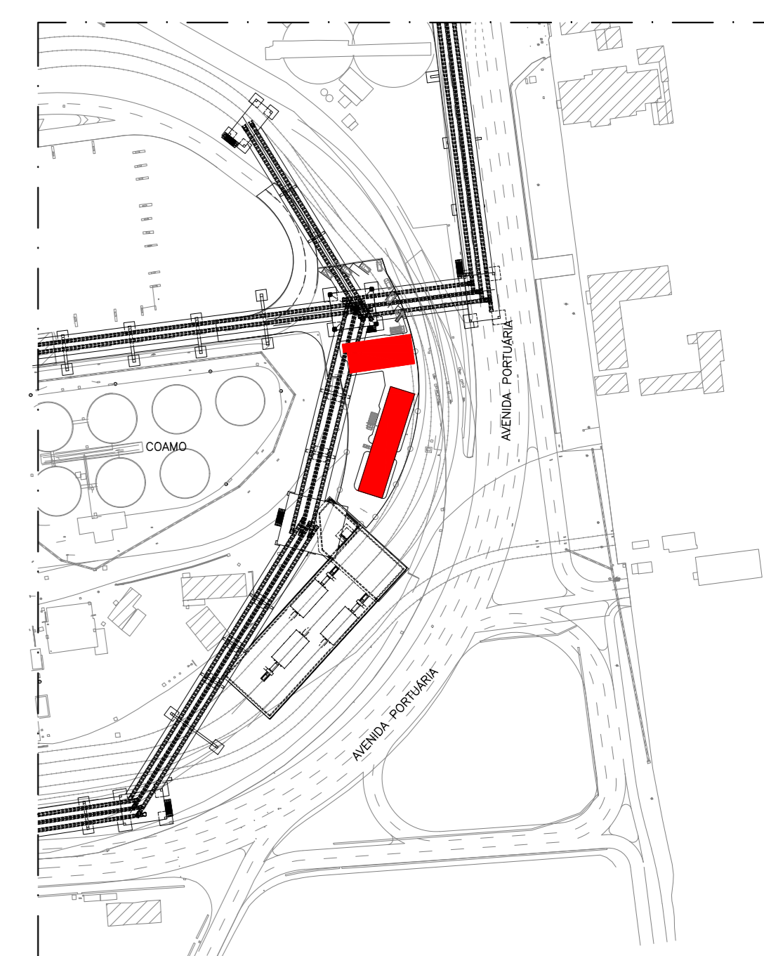
PLANTA SITUAÇÃO 5/1
